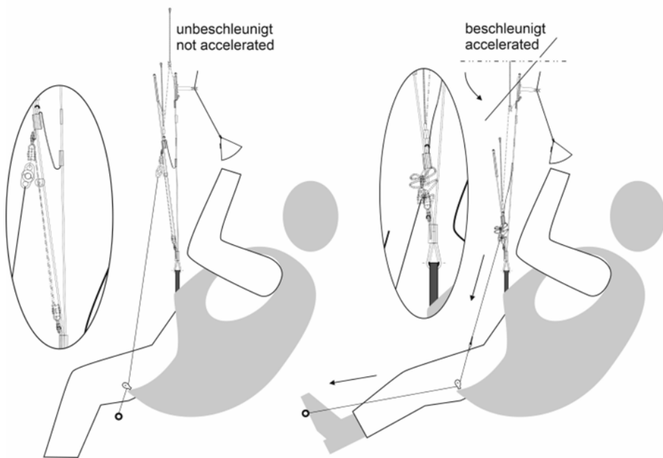
Fig 6 Come lavora il sistema di velocità sulla LIBRA RS.
