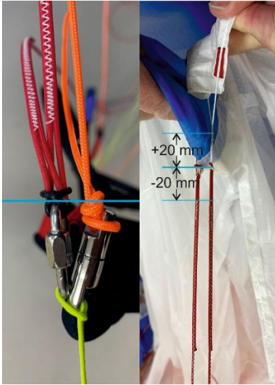
Fig. 9 punto di misurazione veloce per i freni
